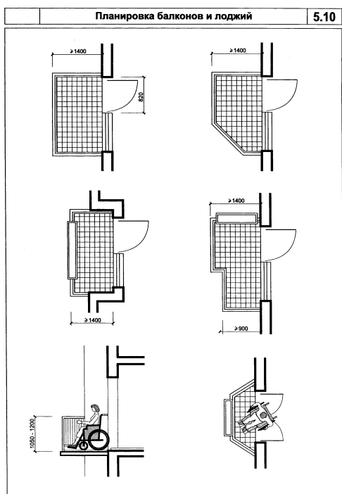
"Рисунок 5.10. Планировка балконов и лоджий"
