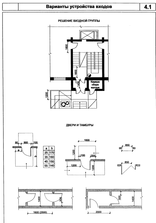
"Рисунок 4.1. Варианты устройства входов",
