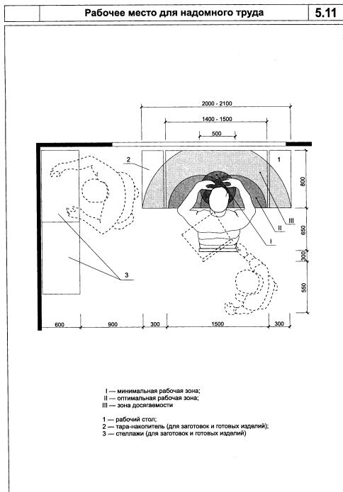
"Рисунок 5.11. Рабочее место для надомного труда"
