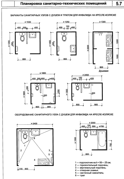
"Рисунок 5.7. Планировка санитарно-технических помещений",
