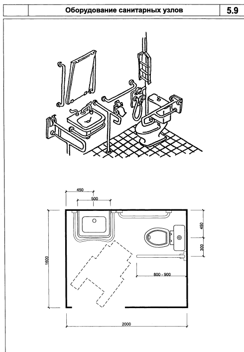
"Рисунок 5.9. Оборудование санитарных узлов"
