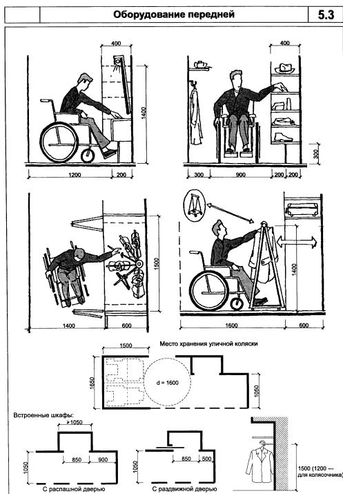
"Рисунок 5.3. Оборудование передней"
