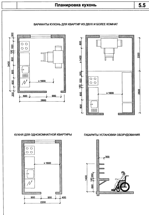
"Рисунок 5.5. Планировка кухонь",
