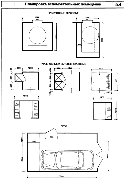
"Рисунок 5.4. Планировка вспомогательных помещений"
