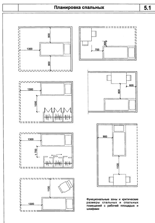
"Рисунок 5.1. Планировка спальных"
